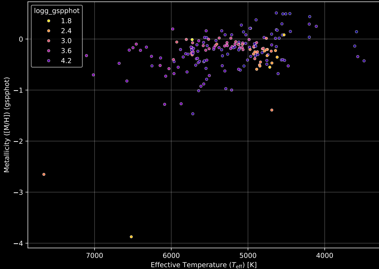
APOGEE DR17 Field: [K2_C6_321+50_btx] Stellar Population Parameters (n= 189)
